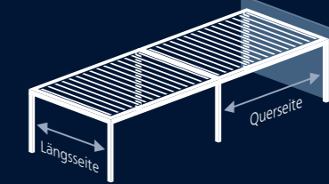
Kopplung in Querrichtung (Anlagen voreinander an der Wand) max. 24 Meter
