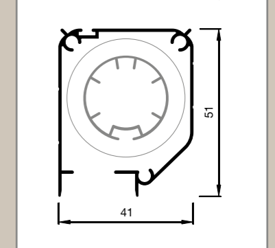
Abdeckung 4151 FR
